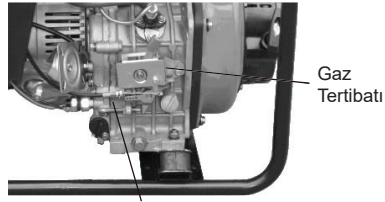
Yakıt enjeksiyon (devir)sınırlama civatası
